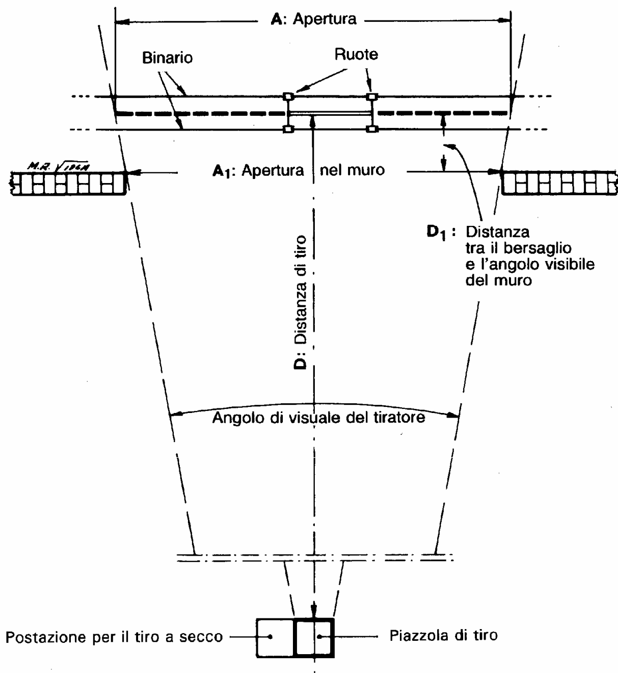
Stand di tiro per Bersaglio Mobile
